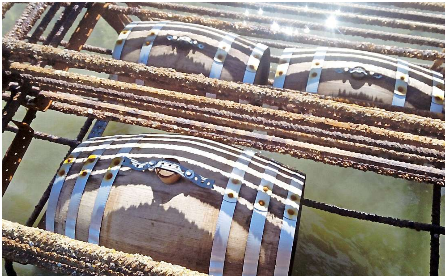
Eine Konstruktion Marke Eigenbau verhindert, dass die Fässer mit dem kostbaren Inhalt abgetrieben werden.
